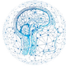
Inteligencia Artificial
